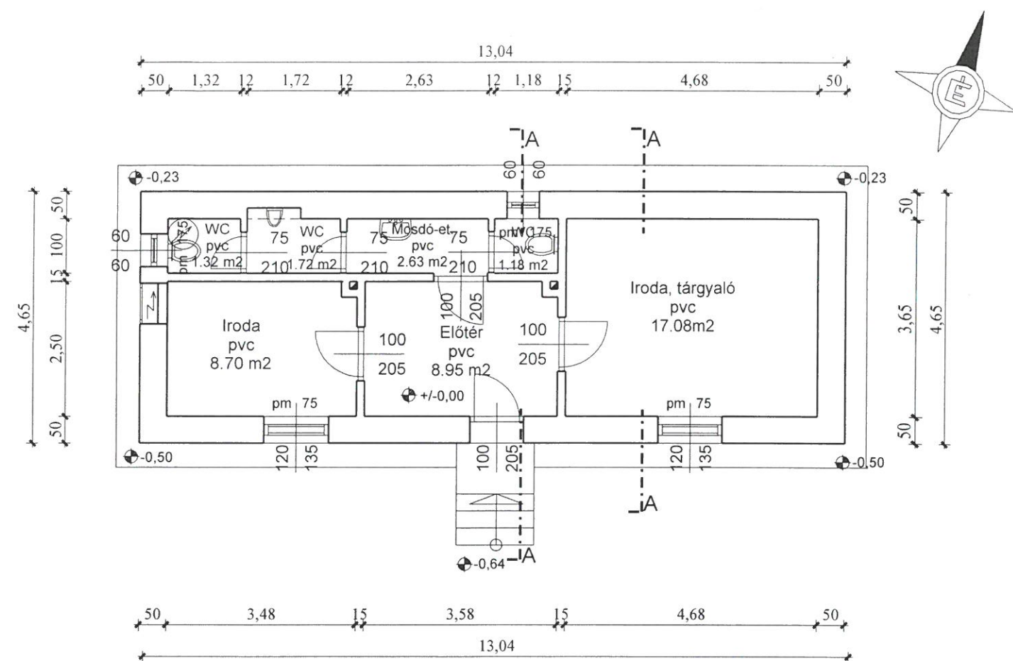
FELMÉRÉSI ALAPRAJZ M=1:100
