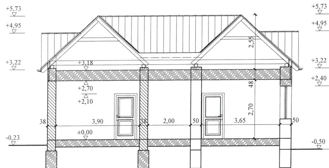
A - A METSZET M=1:100
