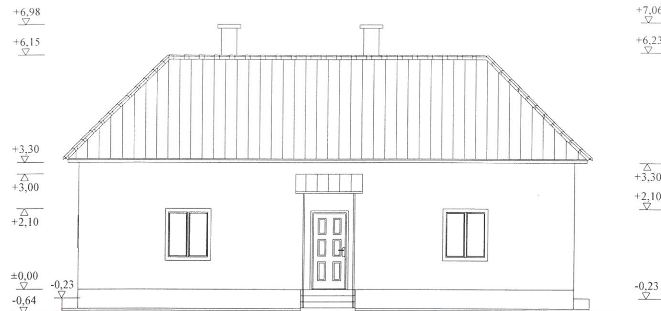
FELMÉRÉSI D-i HOMLOKZAT M=1:100
