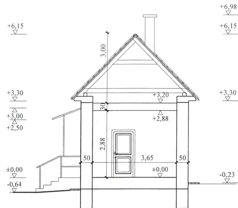
FELMÉRÉSI A-A METSZET M=1:100
