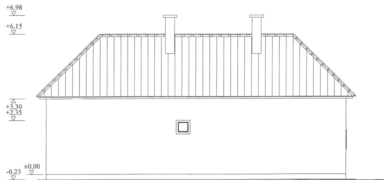
FELMÉRÉSI É-i HOMLOKZAT M=1:100
